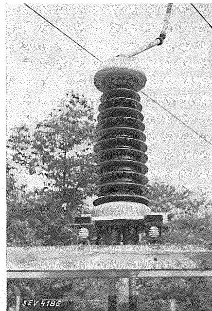
Fig. 6. Ansicht eines 150 kV-Kabelendverschlusses in Lavorgo, mit anschliessendem Mannitwiderstand (oben).
