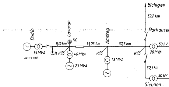
Fig. 3. Prinzipschema des beobachteten 150 kV-Netzes. K Klydonographen-Meßstation. KO Kathodenstrahl-Oszillographen-Station. — Mit Bodenseil ausgerüstete Leitungsstrecke.
