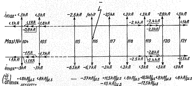
Wie Fig. 20, aber zu Störfall b).
