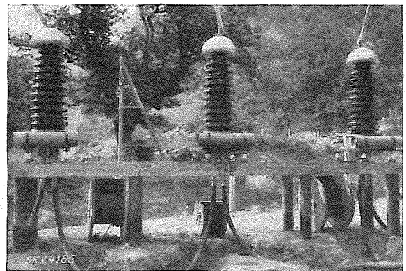
Fig. 5. Ansicht der drei Spannungsteiler für 150 kV in Lavorgo.
