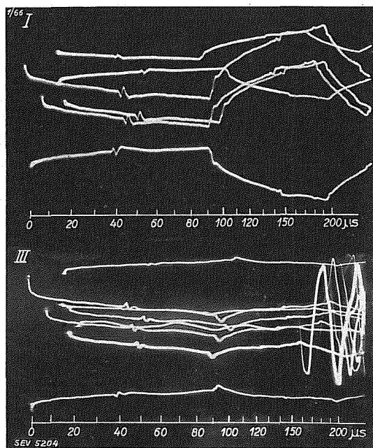
Fig. 25. Oszillogramm zum Blitzstörfall e).
