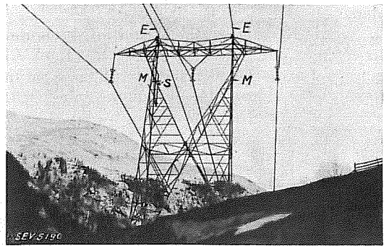
Fig. 11. Bild eines mit «Stahlstäbchen» und Steilheitsmesser ausgerüsteten Tragmastes.
