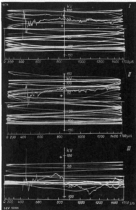
Fig. 27. Oszillogramm zum Blitzstörfall g).
