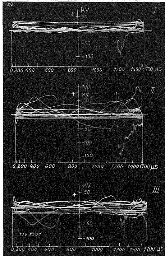
Fig. 28. Oszillogramm zum Blitzstörfall h).
