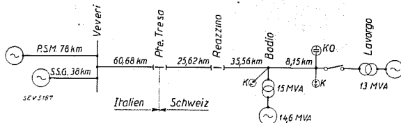
Fig. 4. Prinzipschema des beobachteten 80 kV-Netzes. K Klydonographen-Meßstation. KO Kathodenstrahl-Oszillographen-Station.
