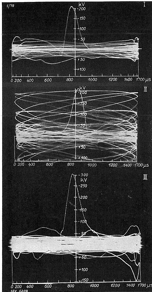
Fig. 29. Oszillogramm zum Blitzstörfall i).
