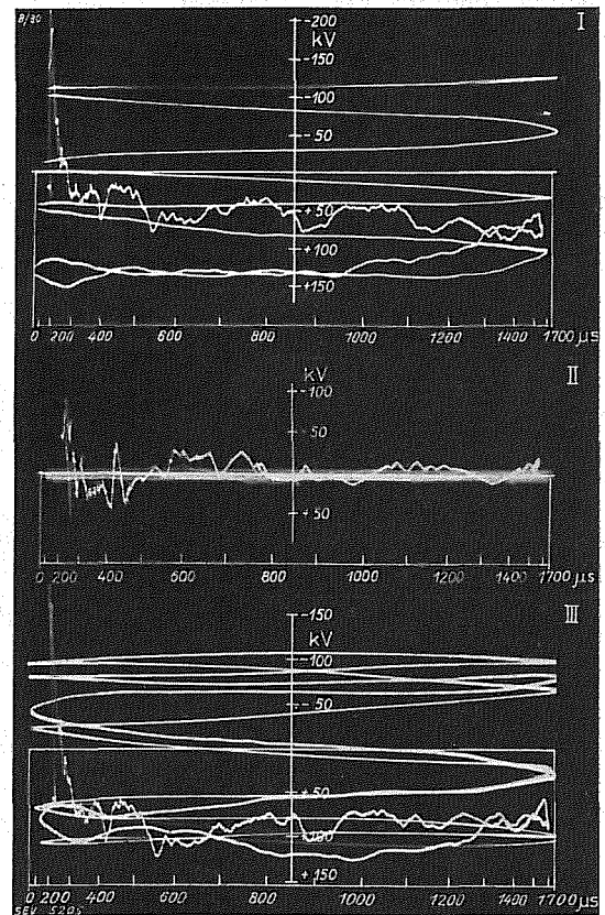
Fig. 26. Oszillogramm zum Blitzstörfall f).
