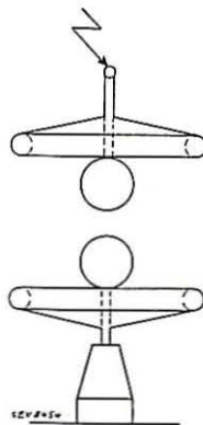
Fig. 4. Geschirmte Kugelfunkstrecke.
