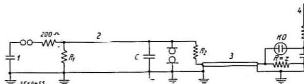
Fig. 5. Schema der Messungen in Gösigen. 1 Stossgenerator. 2 Wellenleitung 1 km. 3 Messkabel. f Schubspannung.
