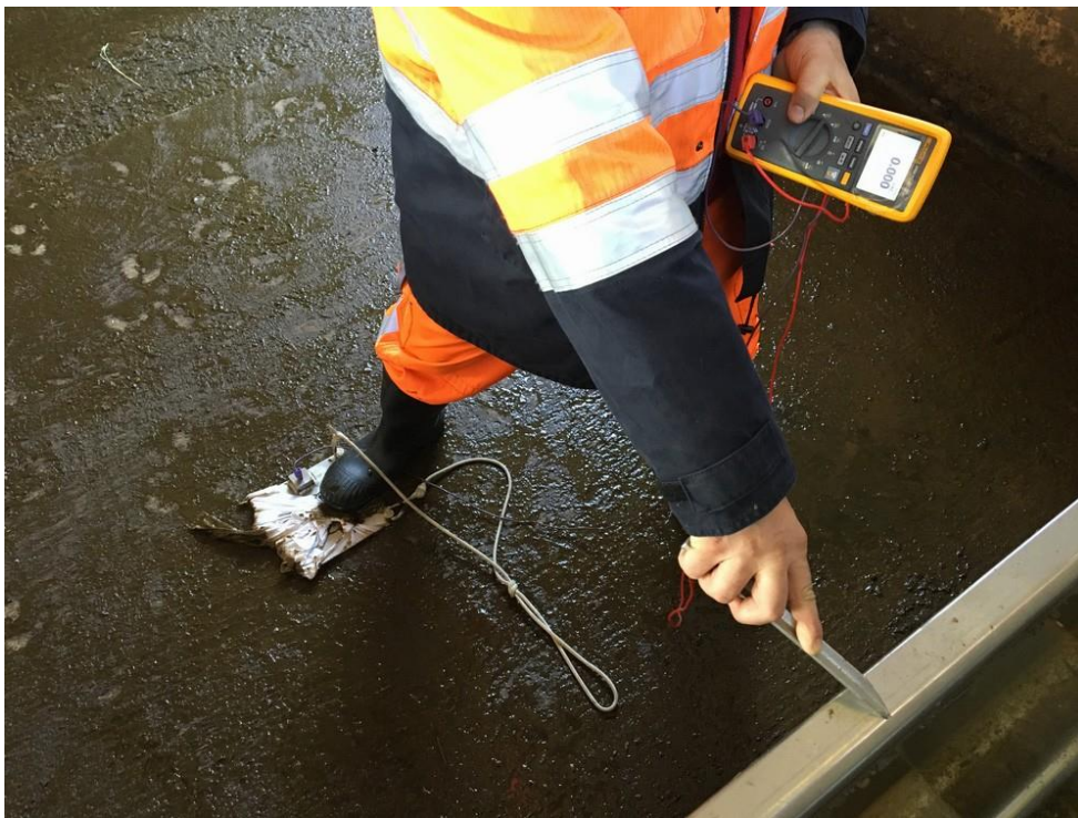
Bild 2 Messung der Wechselspannungsdifferenz zwischen der Standfläche eines Rinds und einer metallischen Tränke. Einfache Möglichkeit zur Kontaktierung des Betonbodens mittels einer Metallplatte, die in einen nassen Lappen eingehüllt wurde. Der Abstand bei dieser Messung entspricht etwa jenen zu den Vorderbeinen.
