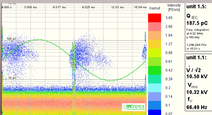
Mesure de décharges partielles lors d'un test de tension
