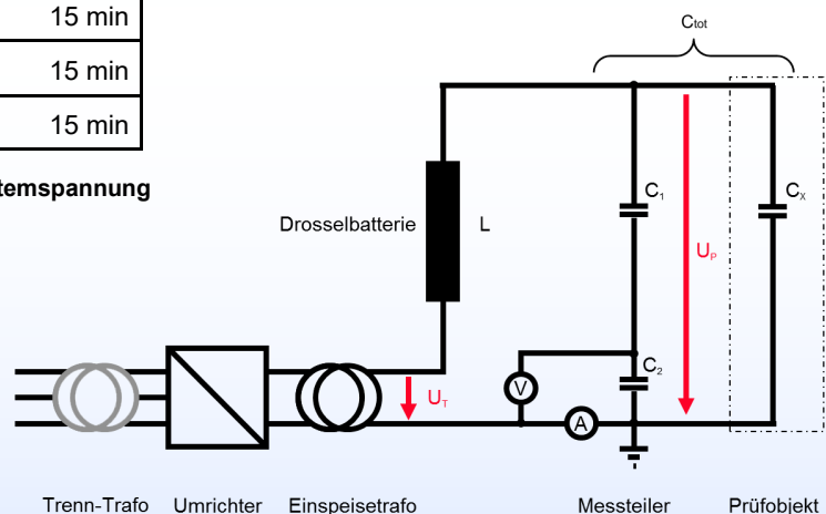
Schema der Serie-Resonanz-Anlage
